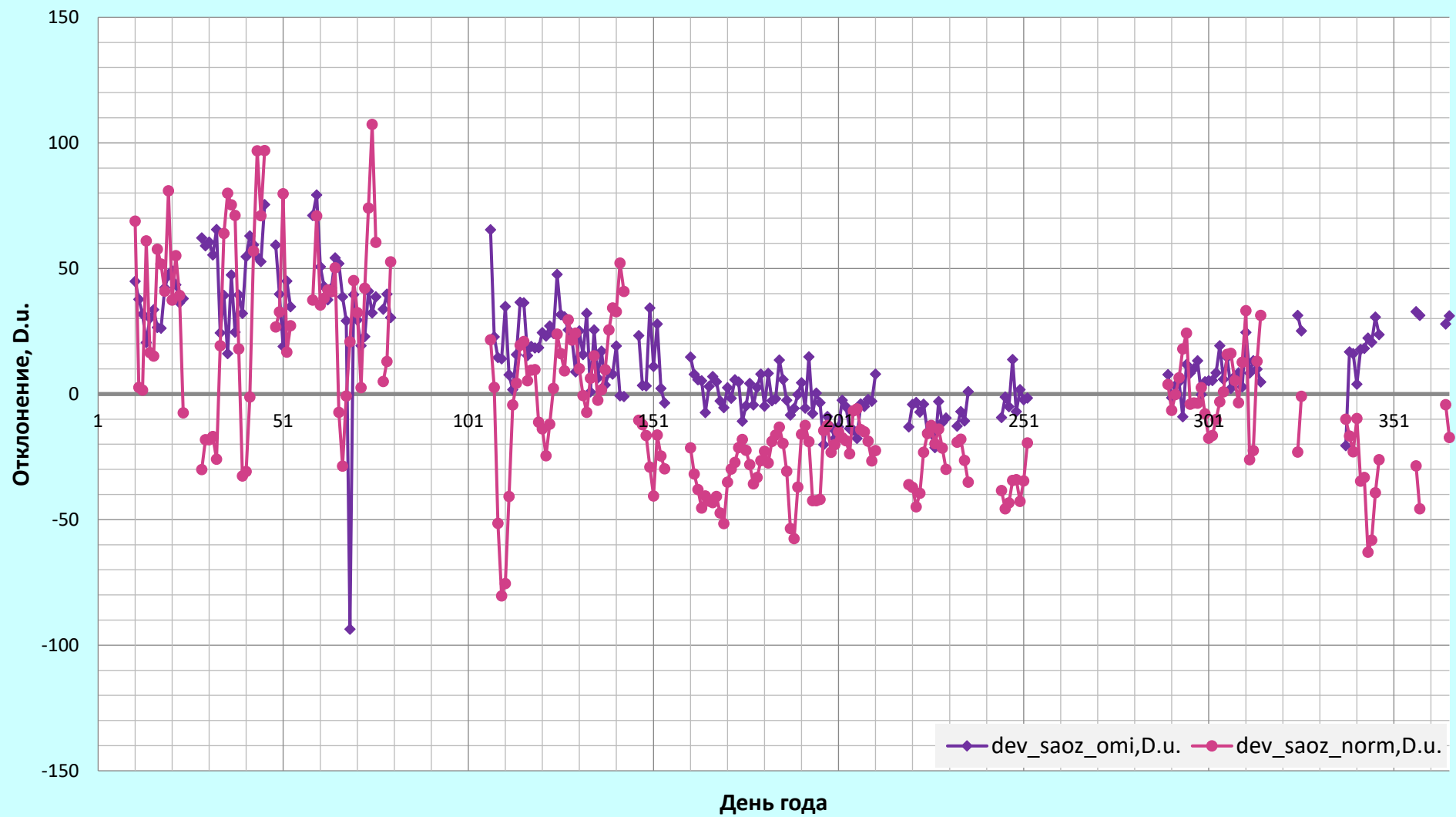
Абсолютные отклонения (D.u.) данных наземных измерений ОСО (Mini-SAOZ) от данных спутниковых измерений ОСО (OMI,NASA) и отклонение наземных измерений (Mini-SAOZ) от климатических норм для ст.Долгопрудный, 1 января - 31 декабря 2020 года.
