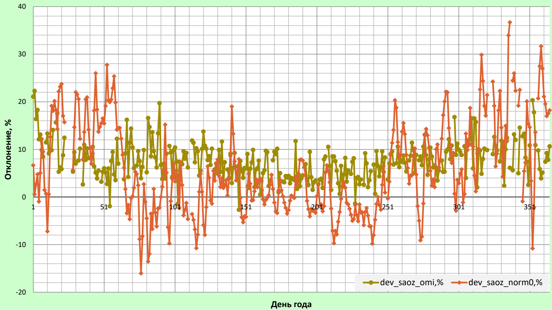
Отклонения (%) данных наземных измерений CO 2 (Mini-SAOZ) от данных спутниковых измерений CO 2 (OMI,NASA) и отклонение наземных измерений (Mini-SAOZ) от климатических норм для ст.Иркутск, 1 января - 31 декабря 2018 года.
