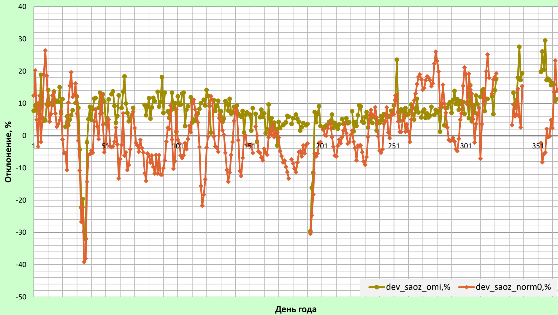
Отклонения (%) данных наземных измерений OCO (Mini-SAOZ) от данных спутниковых измерений OCO (OMI,NASA) и отклонение наземных измерений (Mini-SAOZ) от климатических норм для ст.Иркутск, 1 января - 31 декабря 2017 года.
