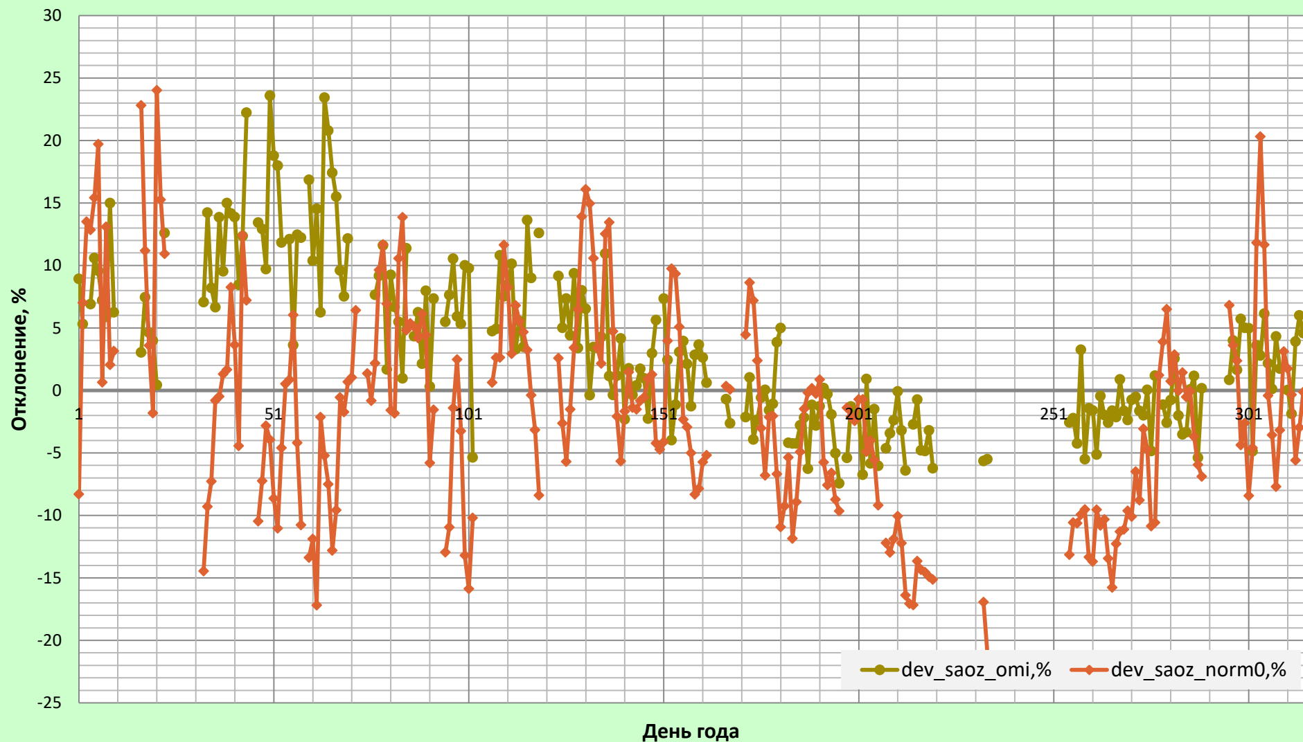
Отклонения (%) данных наземных измерений \text{CO}_2 (Mini-SAOZ) от данных спутниковых измерений \text{CO}_2 (OMI,NASA) и отклонение наземных измерений (Mini-SAOZ) от климатических норм для ст.Долгопрудный, 1 января - 11 ноября 2017 года.
