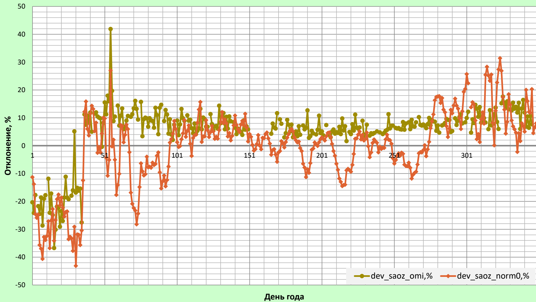
Отклонения (%) данных наземных измерений OCO (Mini-SAOZ) от данных спутниковых измерений OCO (OMI,NASA) и отклонение наземных измерений (Mini-SAOZ) от климатических норм для ст.Иркутск, 1 января - 14 декабря 2016 года.
