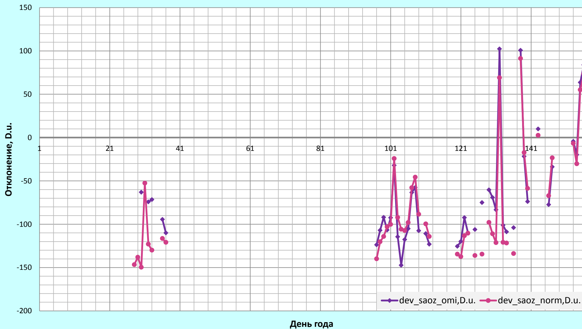
Абсолютные отклонения (D.u.) данных наземных измерений ОСО (Mini-SAOZ) от данных спутниковых измерений ОСО (OMI,NASA) и отклонение наземных измерений (Mini-SAOZ) от климатических норм для ст.Жиганск, 1 января - 5 июня 2015 года.
