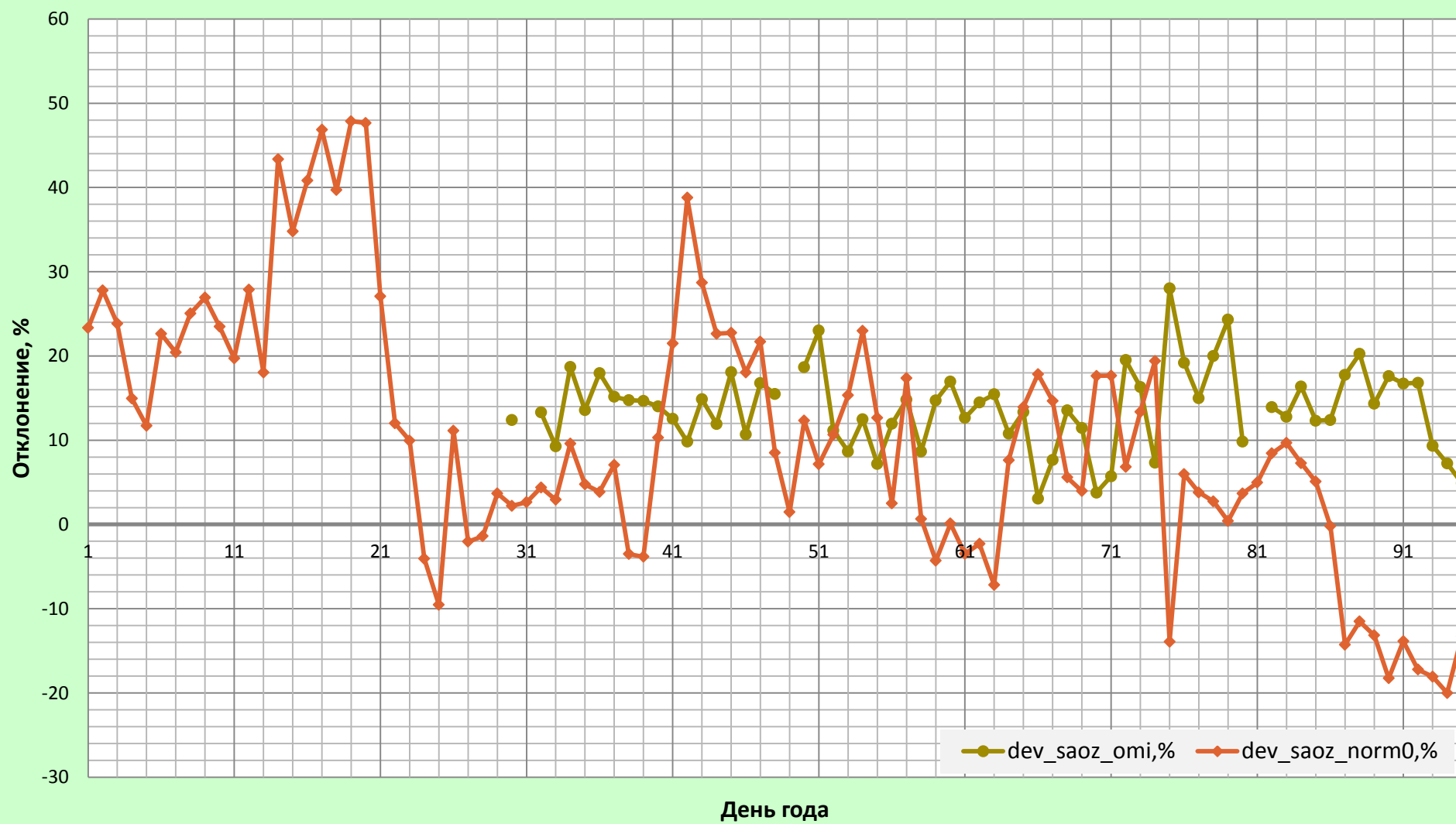
Отклонения (%) данных наземных измерений OCO (Mini-SAOZ) от данных спутниковых измерений OCO (OMI,NASA) и отклонение наземных измерений (Mini-SAOZ) от климатических норм для ст.Салехард, 1 января - 5 апреля 2015 года.
