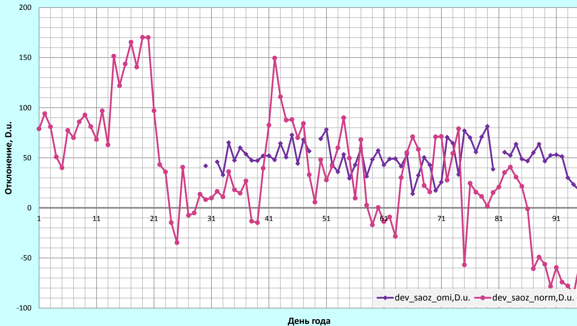
Абсолютные отклонения (D.u.) данных наземных измерений ОО (Mini-SAOZ) от данных спутниковых измерений ОО (OMI,NASA) и отклонение наземных измерений (Mini-SAOZ) от климатических норм для ст.Салехард, 1 января - 5 апреля 2015 года.
