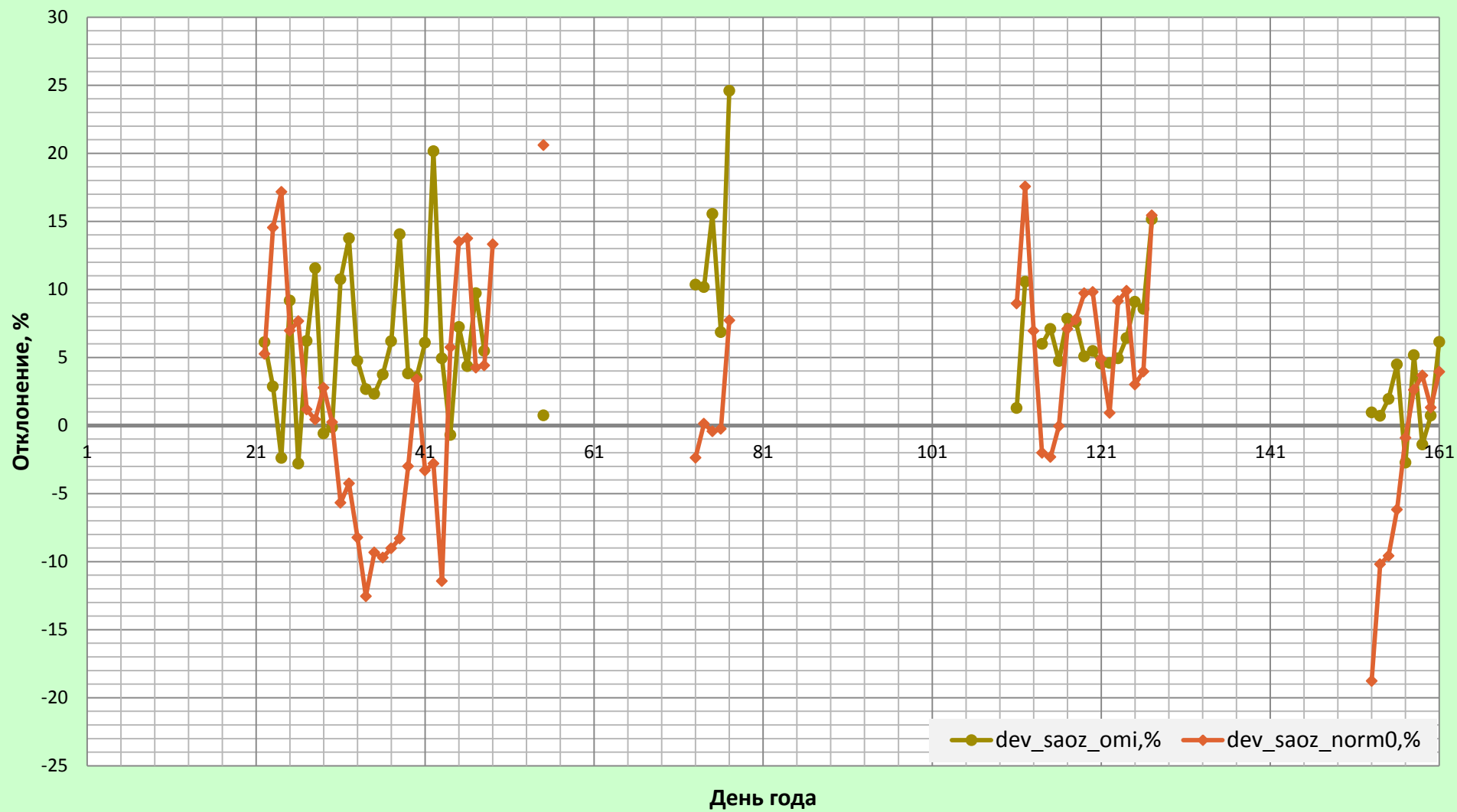
Отклонения (%) данных наземных измерений OCO (Mini-SAOZ) от данных спутниковых измерений OCO (OMI,NASA) и отклонение наземных измерений (Mini-SAOZ) от климатических норм для ст.Анадырь, 1 января - 10 июня 2015 года.
