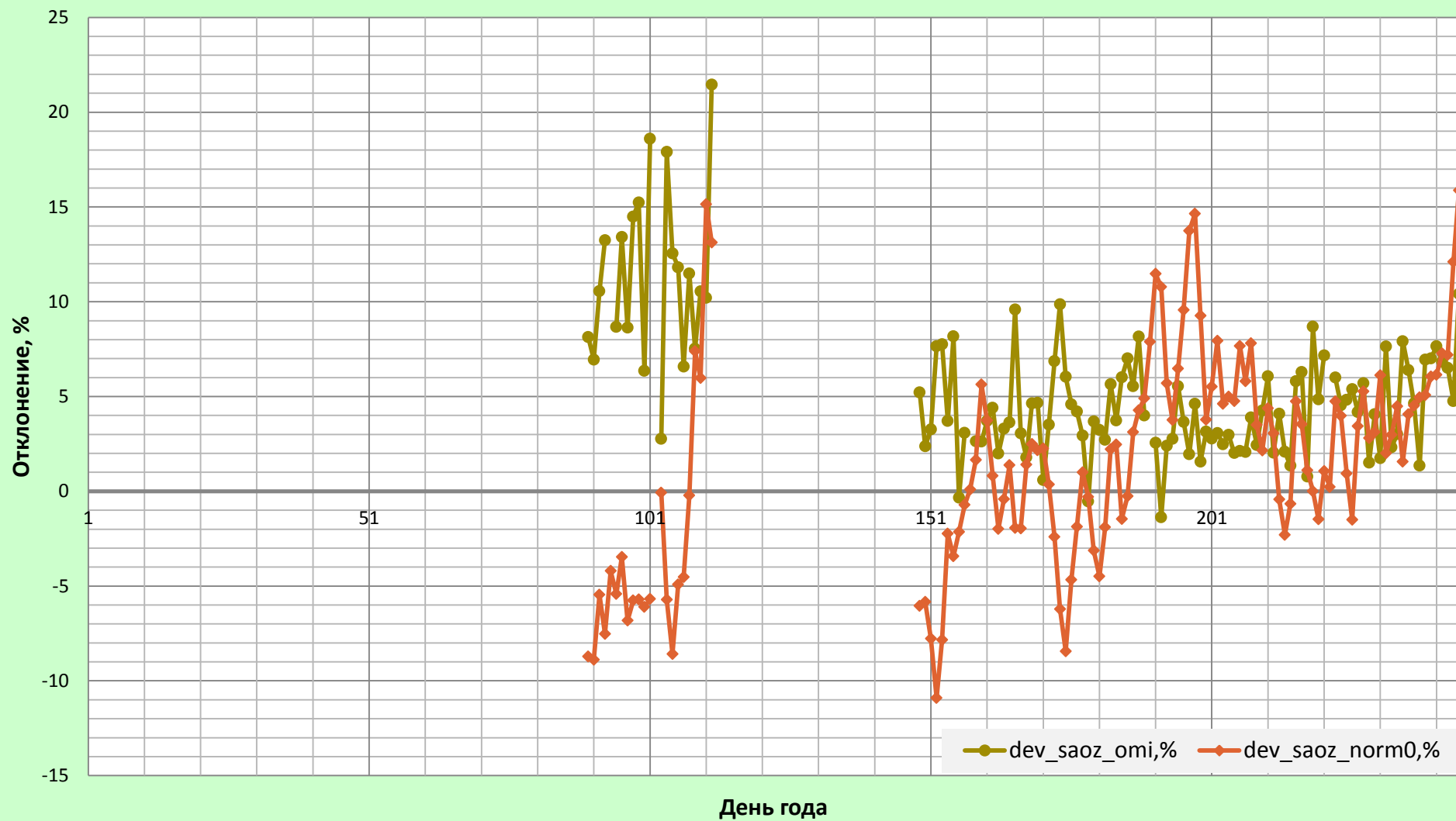
Отклонения (%) данных наземных измерений OCO (Mini-SAOZ) от данных спутниковых измерений OCO (OMI,NASA) и отклонение наземных измерений (Mini-SAOZ) от климатических норм для ст.Салехард, 1 января - 2 сентября 2014 года.
