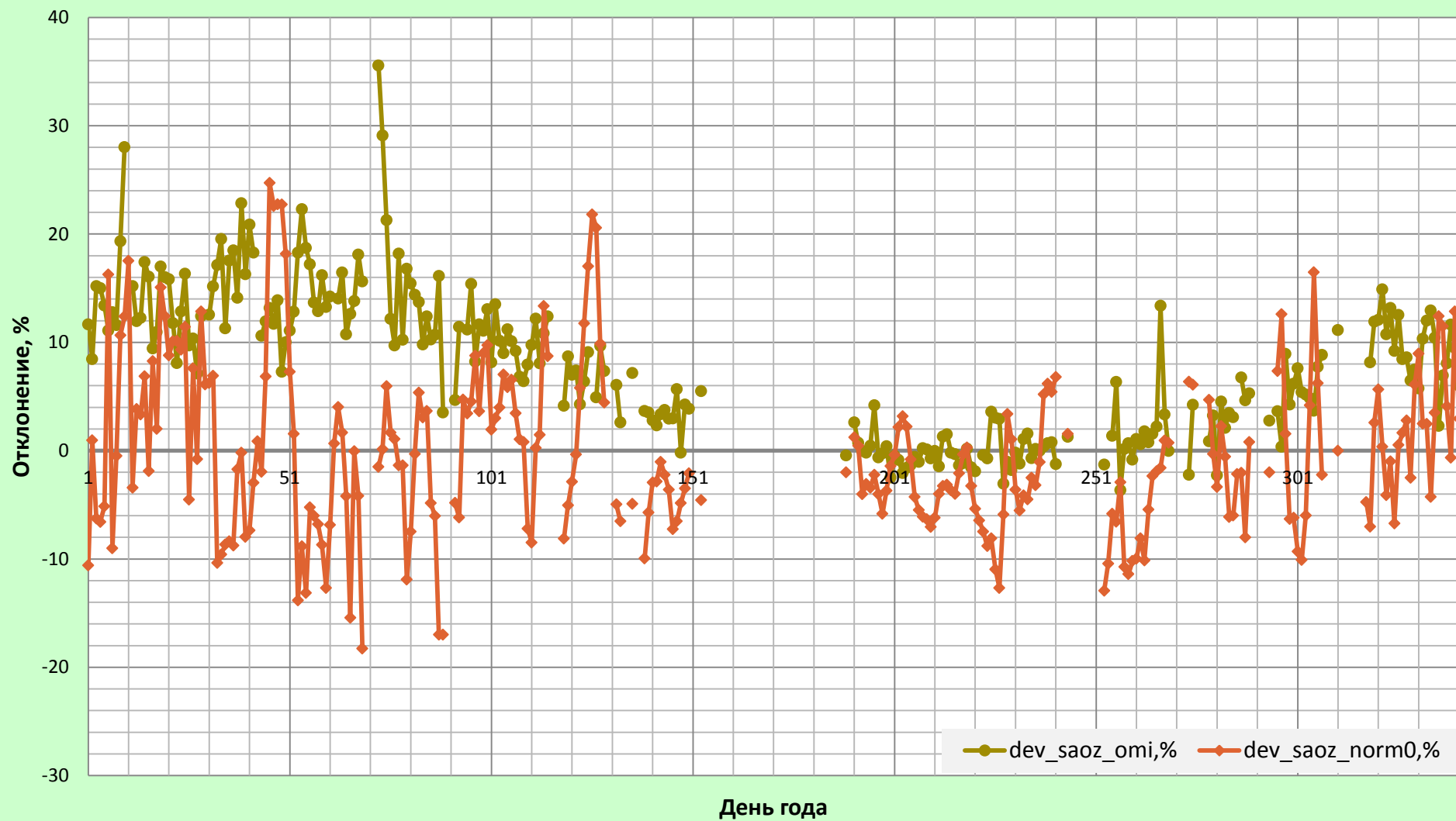
Отклонения (%) данных наземных измерений CO 2 (Mini-SAOZ) от данных спутниковых измерений CO 2 (OMI,NASA) и отклонение наземных измерений (Mini-SAOZ) от климатических норм для ст.Долгопрудный, 1 января - 7 декабря 2014 года.
