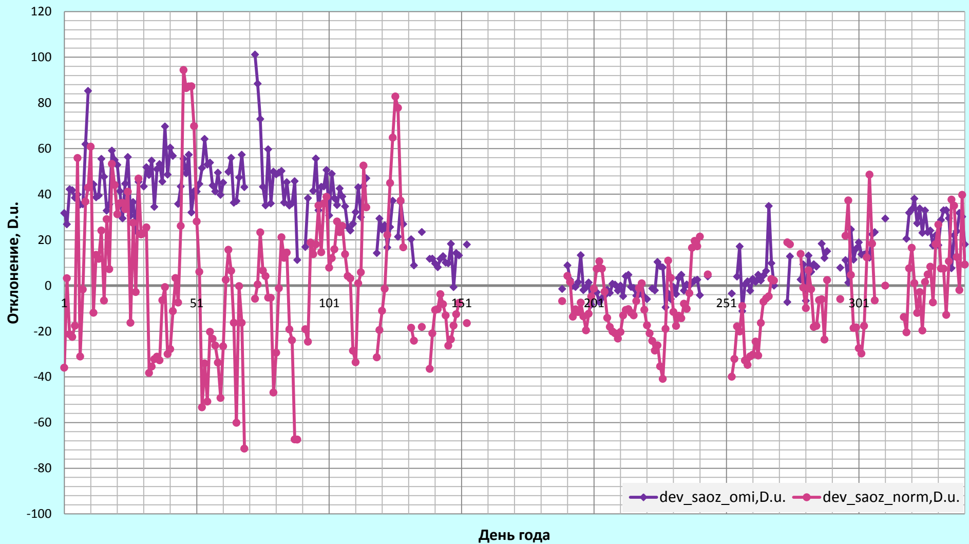
Абсолютные отклонения (D.u.) данных наземных измерений OCO (Mini-SAOZ) от данных спутниковых измерений OCO (OMI,NASA) и отклонение наземных измерений (Mini-SAOZ) от климатических норм для ст.Долгопрудный, 1 января - 7 декабря 2014 года.
